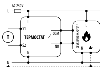
а) Схема на свързване към котел
