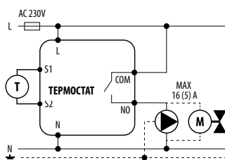
б) Схема на свързване към помпата/задвижката
