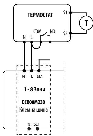
в) Схема на свързване към клемна шина
